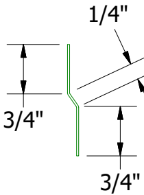
Joggle Cleat
