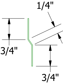
Joggle Cleat
