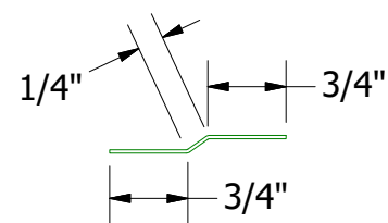
Joggle Cleat
