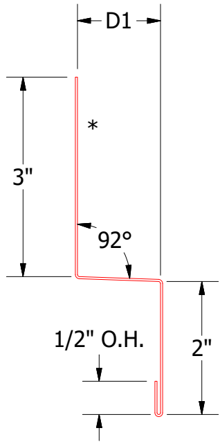
Head Trim DWA550: D1= 1 1/4" DSA550: D1= 2"
