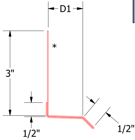
Base Trim DWA661: D1= 1 1/4" DSA661: D1= 2"
