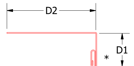
Snap Base DWA119: D1 = 1 1/8", D2 = 3" DSA179: D1 = 1 7/8", D2 = 2 1/4"
