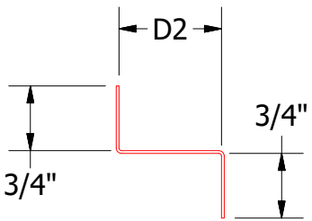
Z Closure D2=1 3/16" D2=1 15/16"
