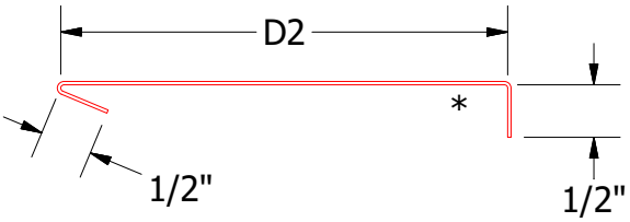
Head Angle Trim DWA690: D2= 4 1/4" DSA690: D2= 5"
