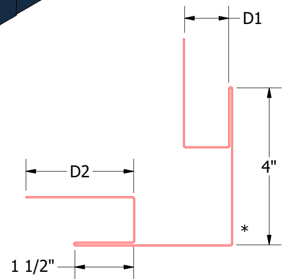
Outside Corner Post DWA602: D1 = 1 1/8", D2 = 2 3/4" DSA602: D1 = 1 7/8", D2 = 3"
