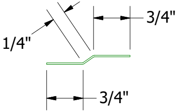
Joggle Cleat
