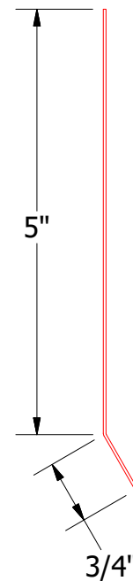
HLA349-Starter Cleat
